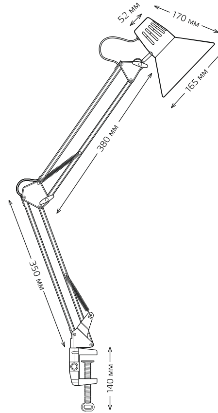
Рис. 1. Размеры светильника
